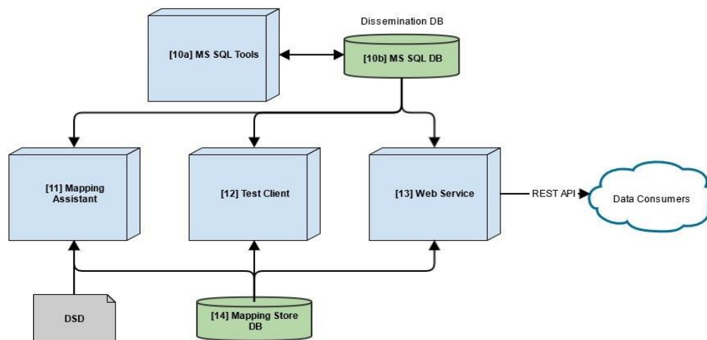
Εικόνα 3: Υποδομή SDMX
