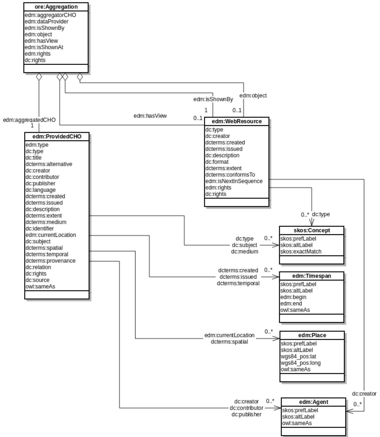
Εικόνα 2. Διάγραμμα κλάσεων του EDM μοντέλου
